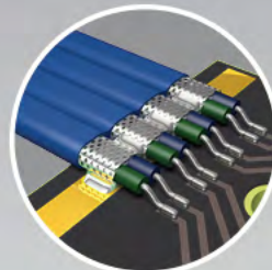
32 AWG Twinax
